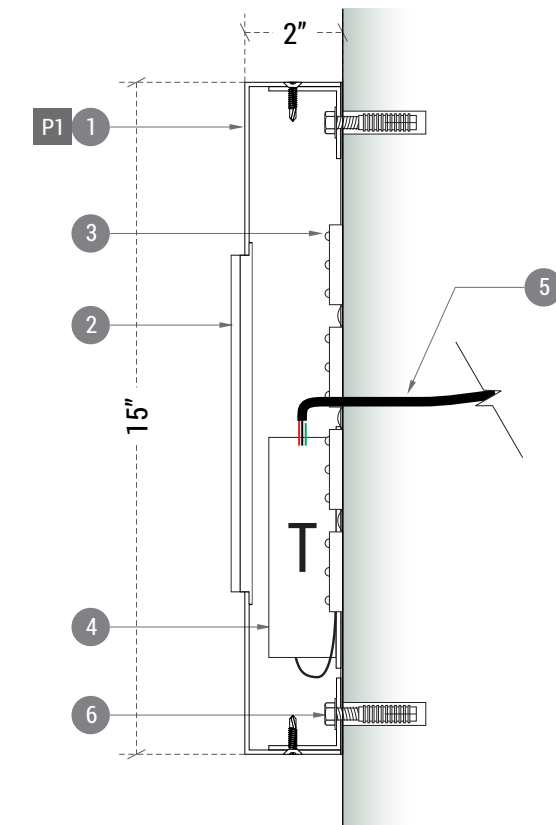
A.1 Section View SCALE: 1:4
