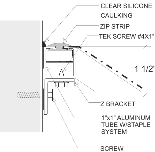
D1 Top /Bottom Connection Detail Scale: NTS
