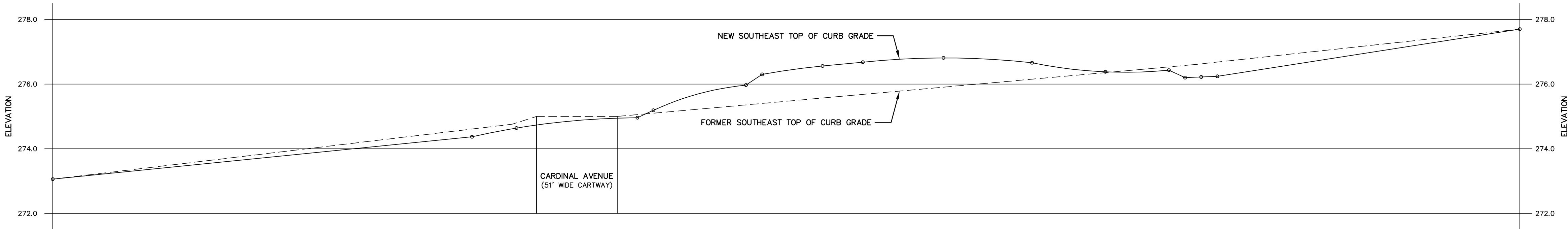
PROFILE VIEW HORIZ. SCALE: 1" = 40' VERT. SCALE: 1" = 2'
