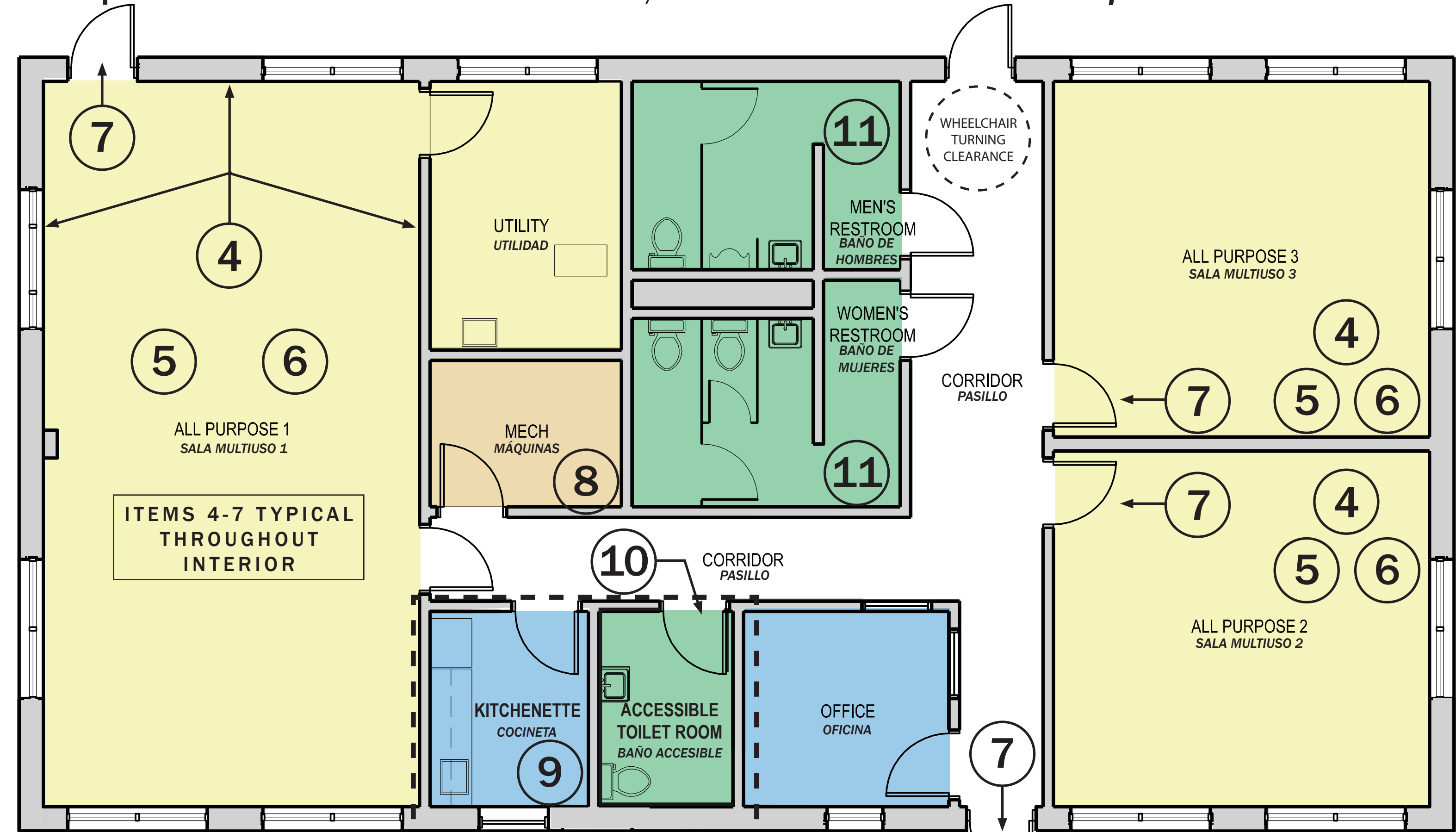
Proposed Plan Plano Propuesto
