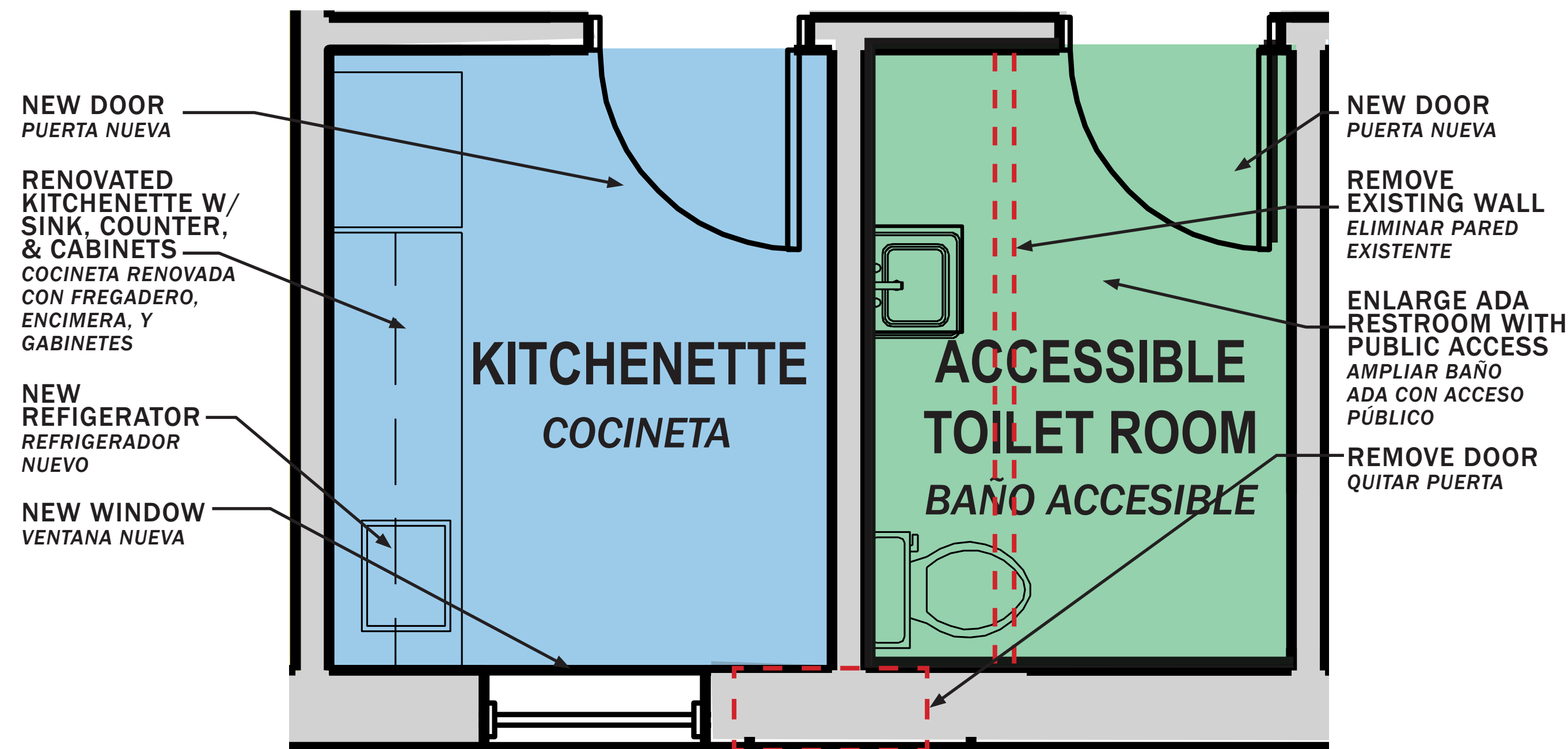
Enlarged Bathroom & Kitchenette Plan Plano de Baño y Cocineta Engrandecida
