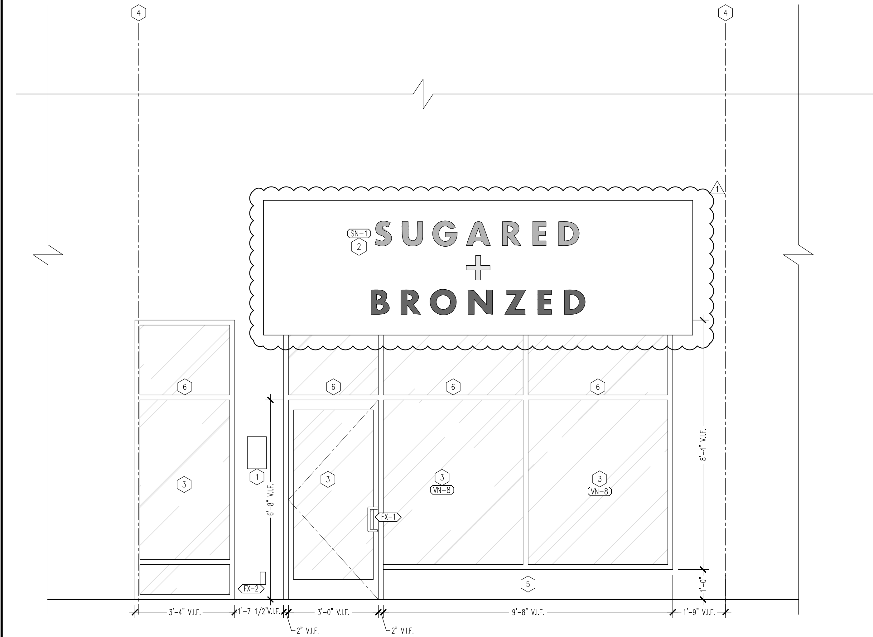
01 EXTERIOR ELEVATION SCALE: 1/2"=1'-0"
