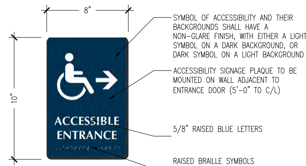
02 H.C. ENTRY SIGN SCALE: N.T.S.
