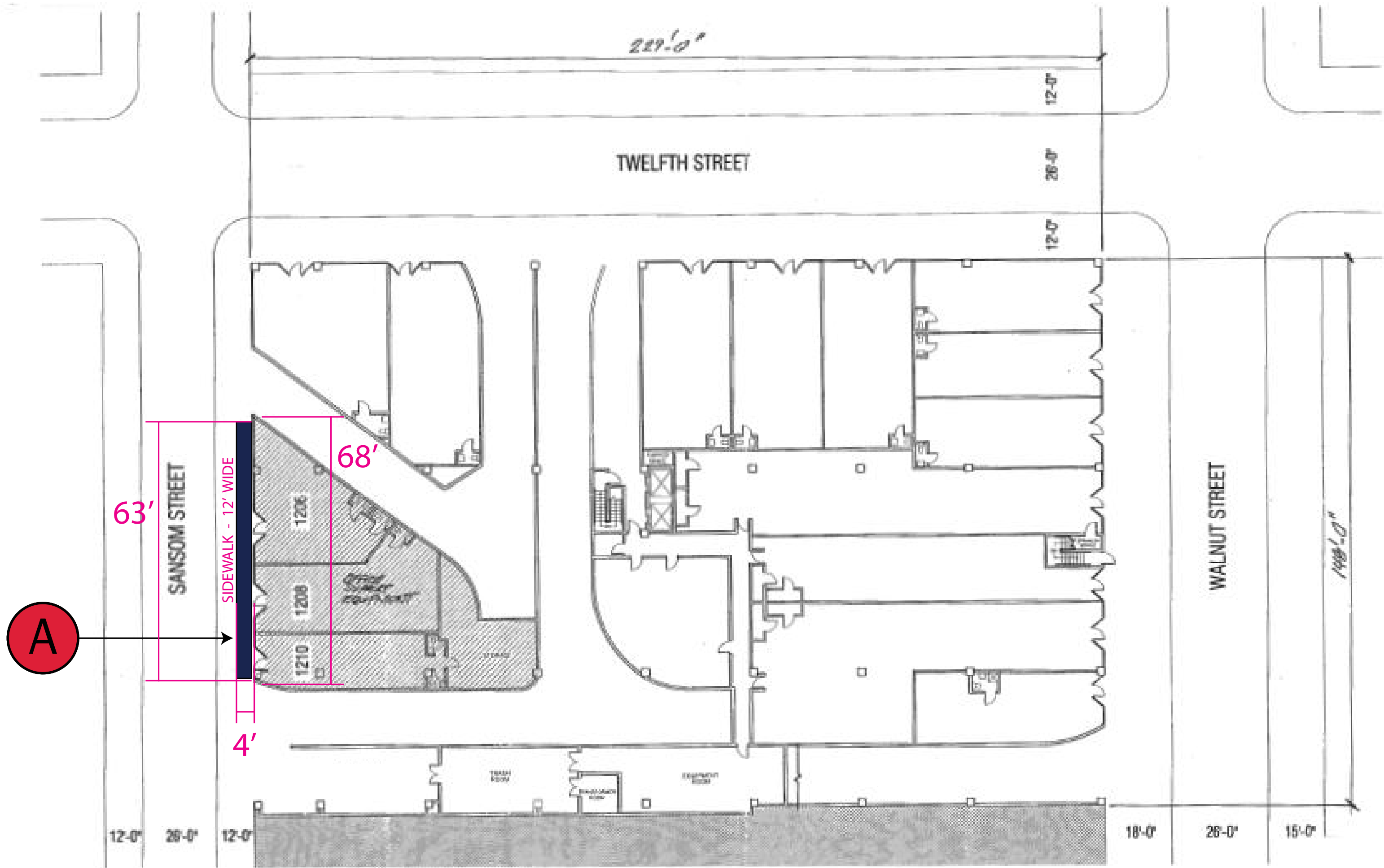
1206, 1208 & 1210 SANSOM TENANT SPACE GROUND FLOOR PLAN / SITE PLAN
