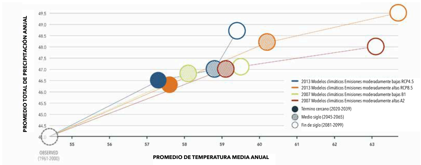
CAMBIOS PROYECTADOS EN LA TEMPERATURA ANUAL PROMEDIO Y LA PRECIPITACIÓN ANUAL, TOTAL EN FILADELFIA, BAJO CUATRO ESCENARIOS DE EMISIONES DE CARBONO
